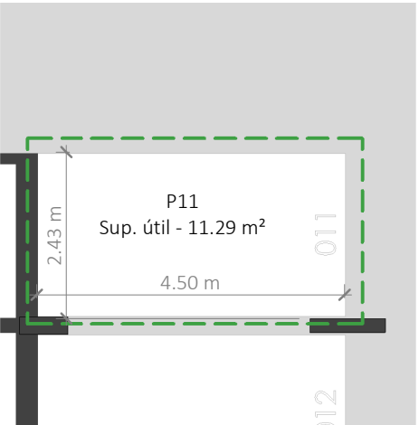
Aparcamiento - Plaza P11 1 : 100 / PARKING - SPOT P11
