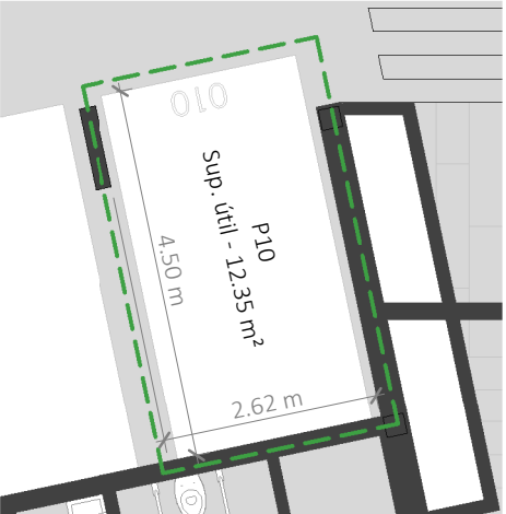
Aparcamiento - Plaza P10 1 : 100 / PARKING - SPOT P10
