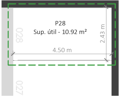
Aparcamiento - Plaza P28 1 : 100 / PARKING - SPOT P28
