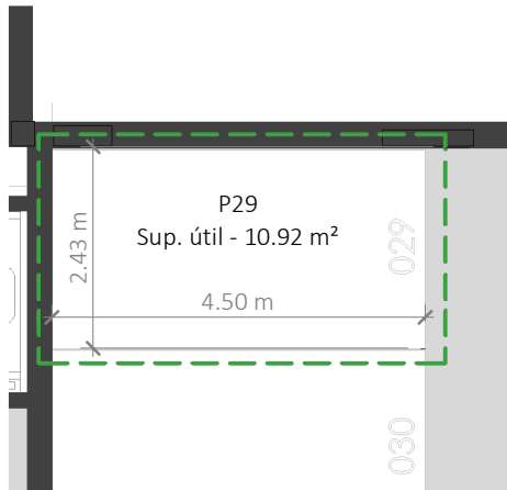
Aparcamiento - Plaza P29 1 : 100 / PARKING - SPOT P29
