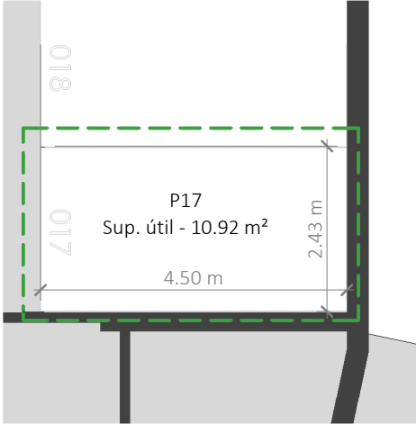
Aparcamiento - Plaza P17 1 : 100 / PARKING - SPOT P17
