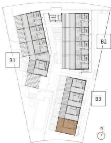
Planta Primera
