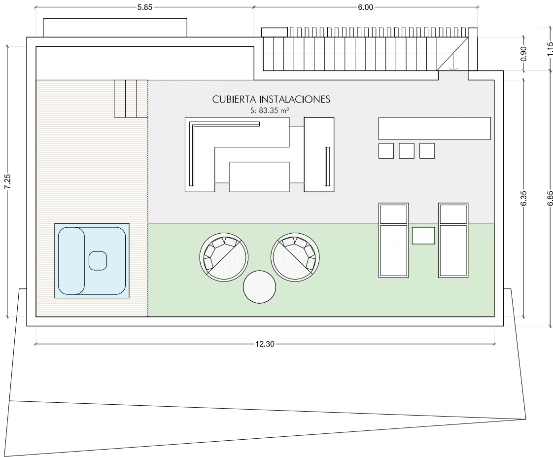
Planta Solarium
