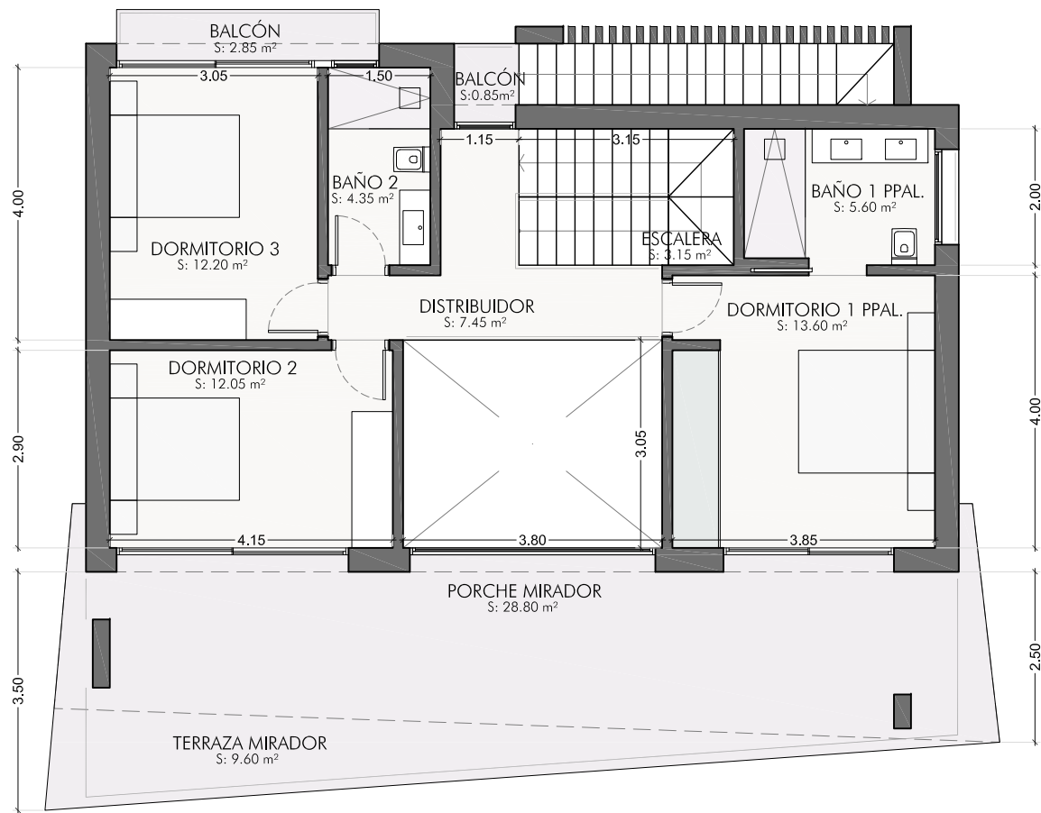
Planta Primera
