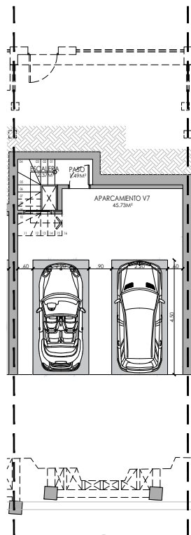
PLANTA SÓTANO T4 V07
