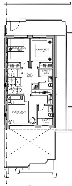
PLANTA ALTA T1.B V04
