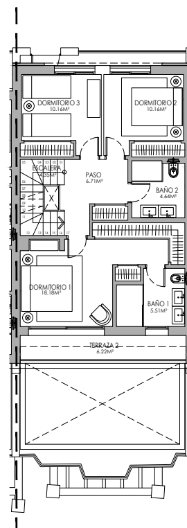
PLANTA ALTA T4 V07
