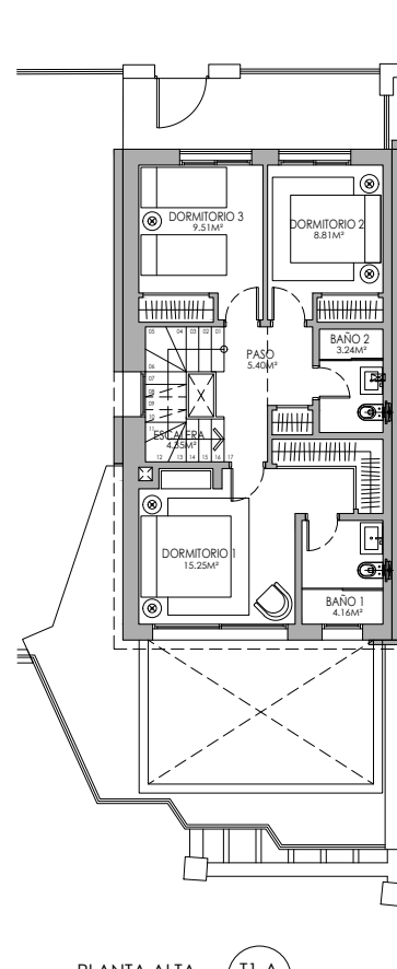
PLANTA ALTA T1-A V01
