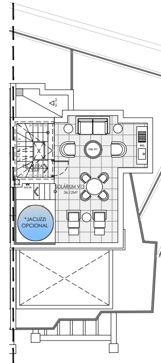
PLANTA SOLÁRIUM T6 V13
