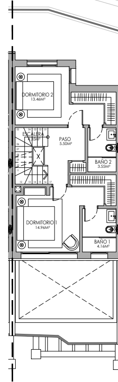
PLANTA ALTA T5 V12
