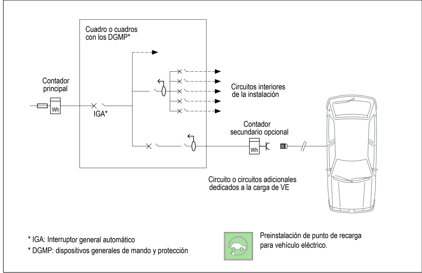
ESQUEMA DE INSTALACIÓN CON CIRCUITO ADICIONAL INDIVIDUAL PARA LA RECARGA DEL VEHÍCULO ELÉCTRICO EN VIVIENDAS UNIFAMILIARES
