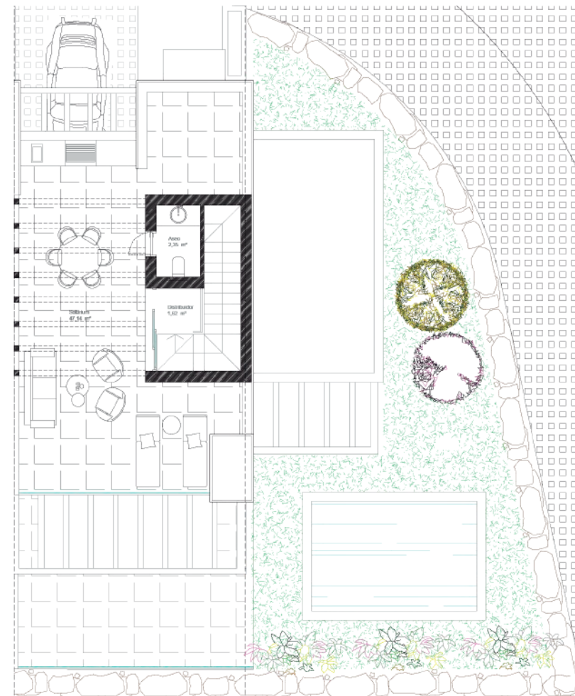
PLANTA 2
