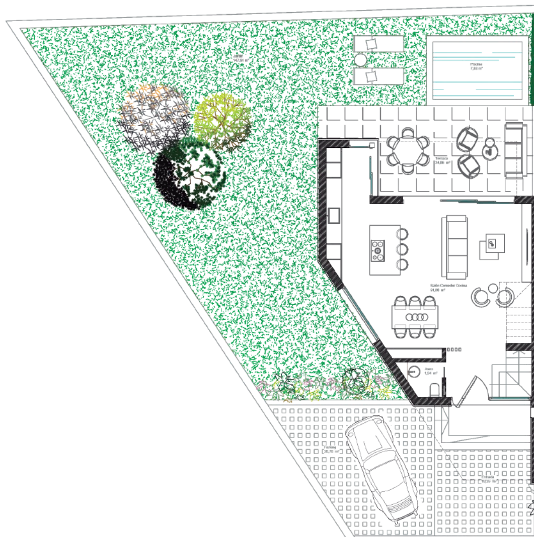
PLANTA BAJA
