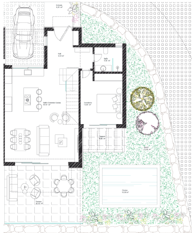
PLANTA BAJA
