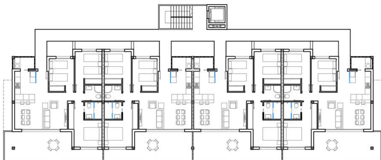
PLANTA PRIMERA
