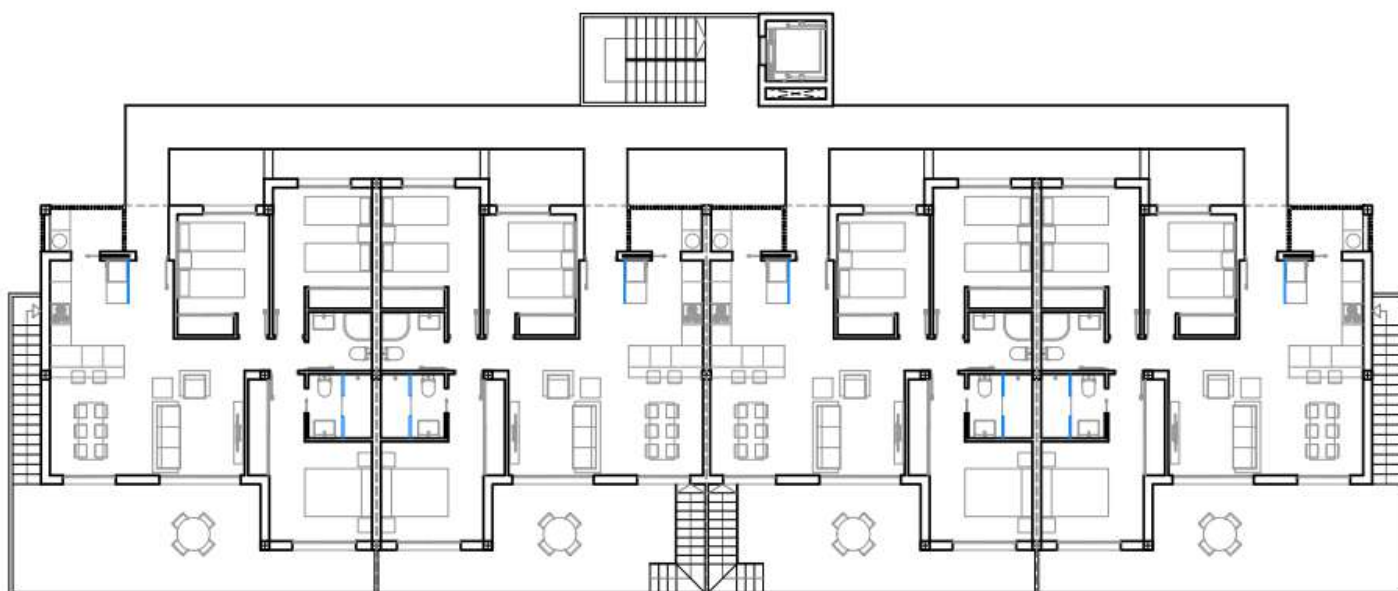
PLANTA ÁTICO
