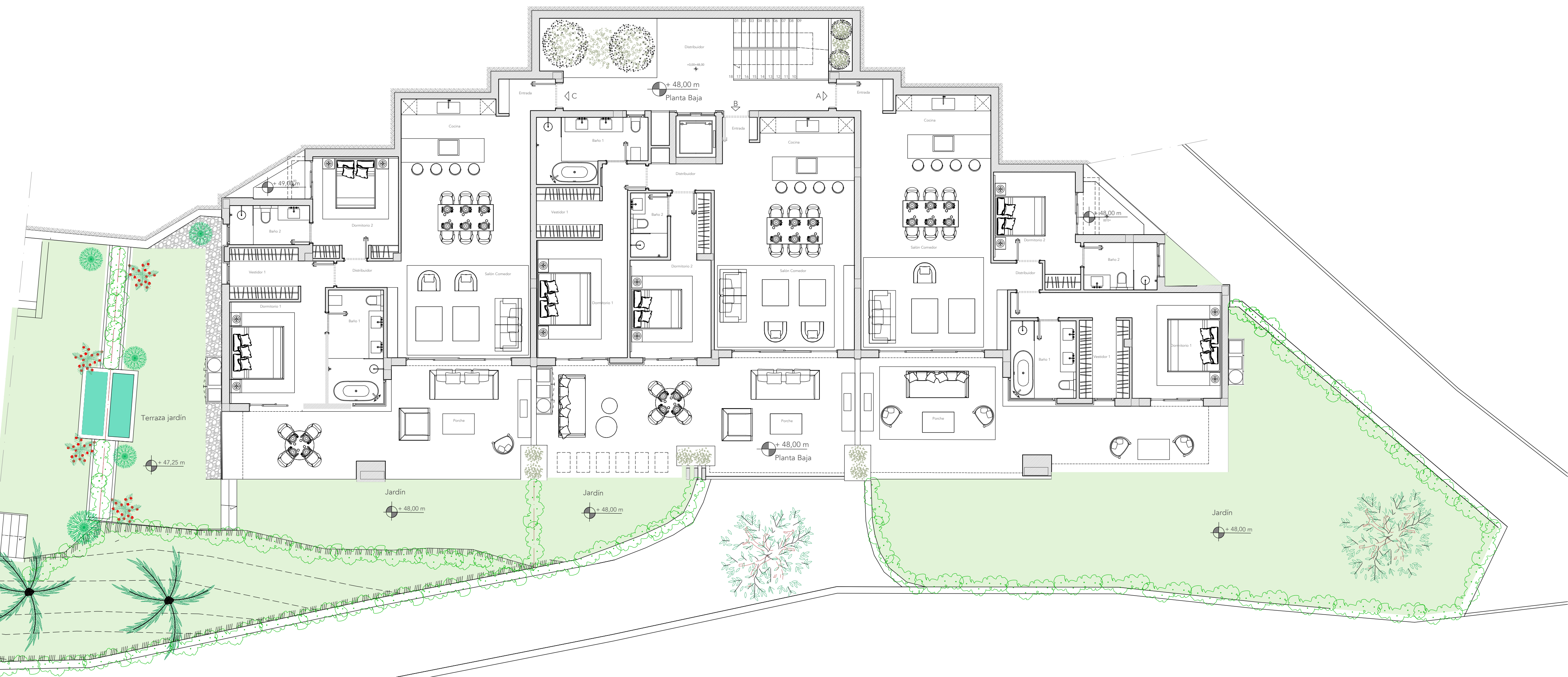
PLANTA BAJA_BLOQ. 2
