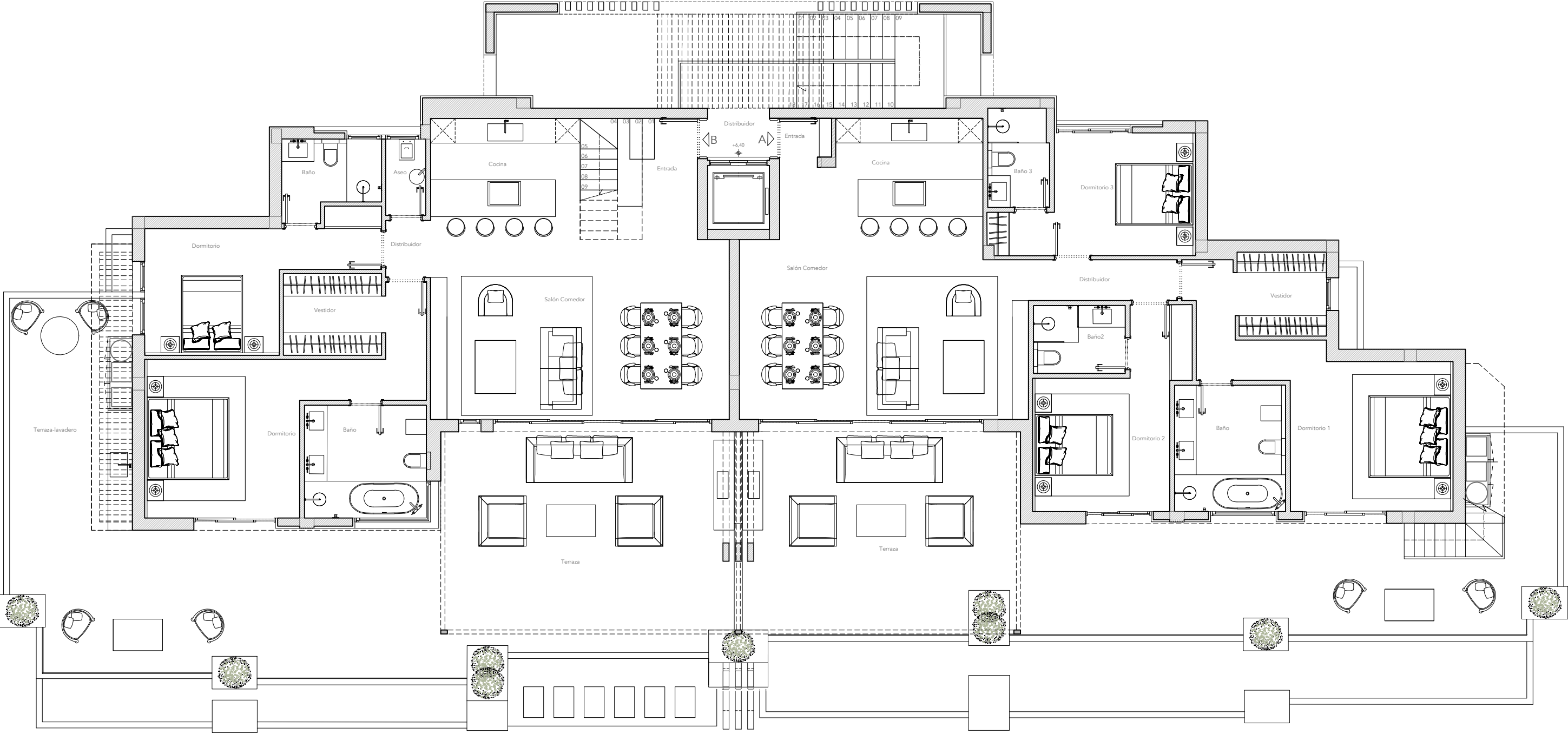
PLANTA SEGUNDA_BLOQ. 2
