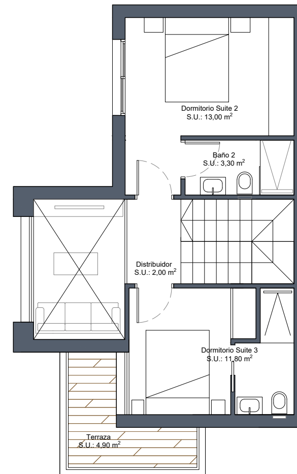
Planta primera
