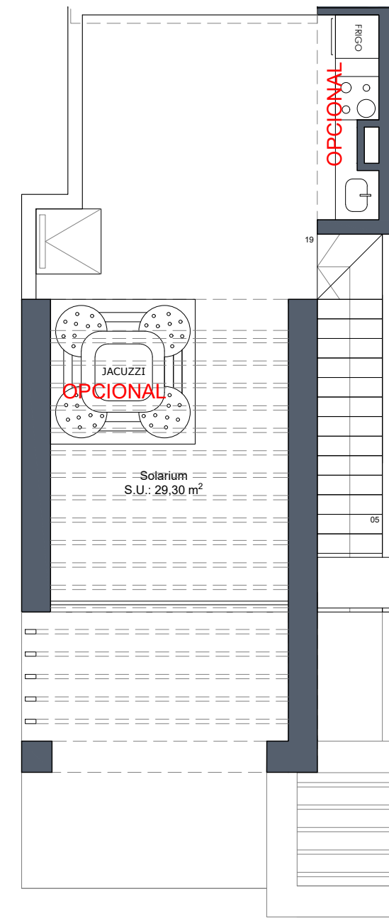
Planta solarium
