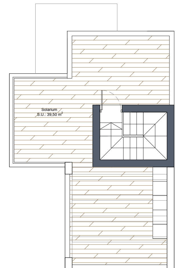
Planta solarium
