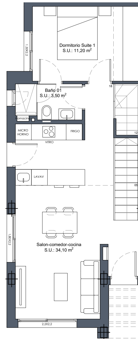
Planta baja
