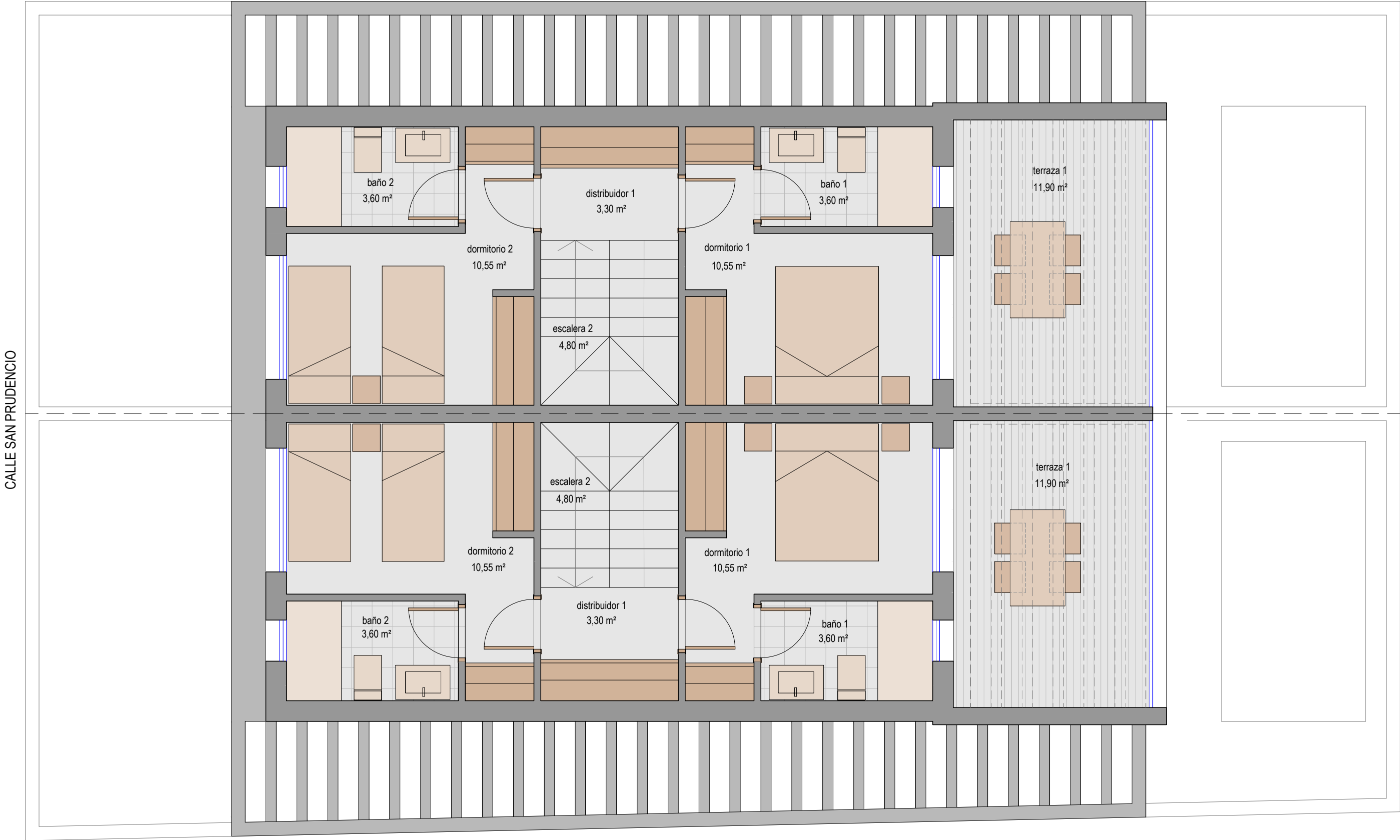
PLANTA PRIMERA
