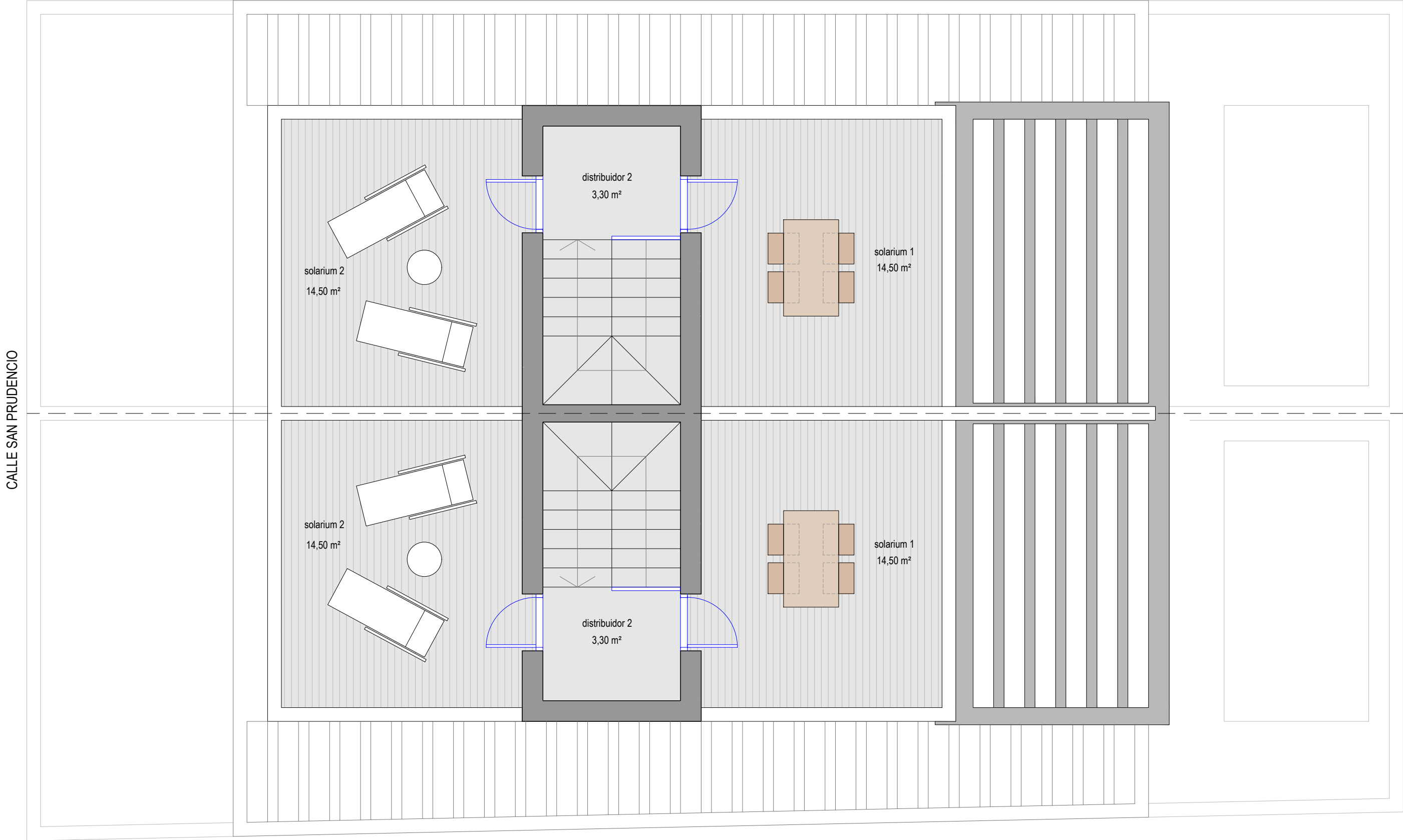
PLANTA TORREÓN
