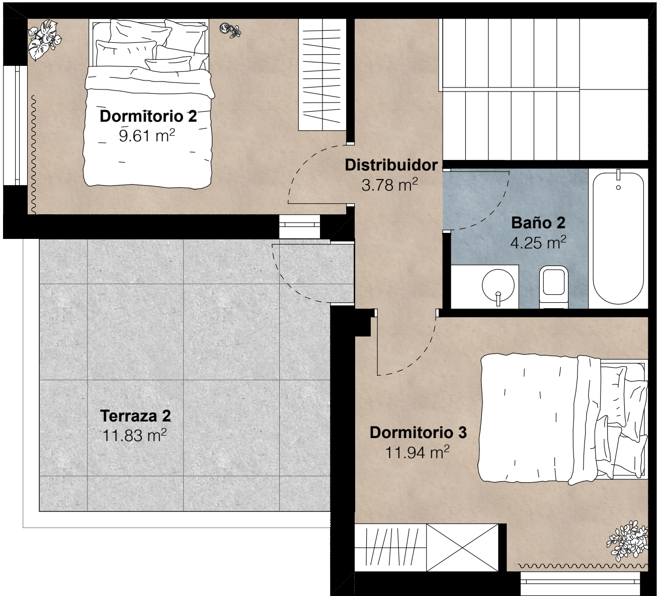
Planta primera
